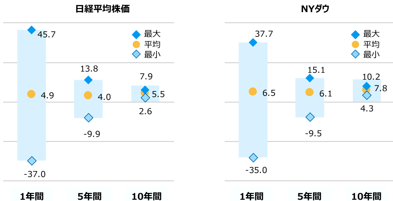
<日経平均株価とNYダウに積立投資した場合の投資期間別の運用リターン（年率、%）> 2003年4月末～2023年4月末
