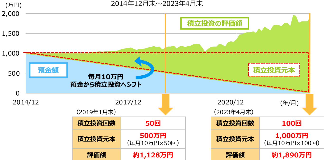
＜預金1,000万円を毎月10万円ずつNYダウへ積立投資した場合の推移＞ 2014年12月末～2023年4月末
